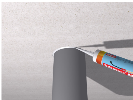
4. Den Ringspalt (max. 5 mm) mit Intumex AN in einer Mindesttiefe von 20 mm verfüllen.
