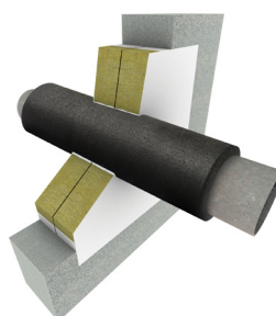
Metallrohr mit K-Flex R90 (25mm dick)
