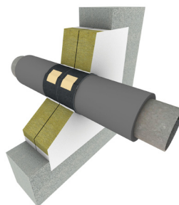
Metallrohr mit brennbarer Dämmung mind. RF2 (cr) mit Intumex® Wrap
