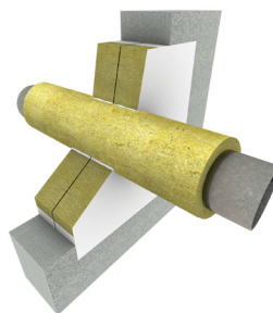
Metallrohr mit nicht brennbarer Dämmung (mind. 40 kg/m 3 , mind. 30 mm dick)
