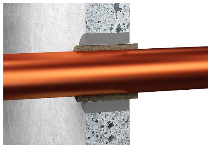
RF1 Ringspaltverschluss einer einzeln geführten Leitung gemäss VKF-Brandschutzrichtlinie 15-15 und VKF-Brandschutzmerkblatt 2004-15.
