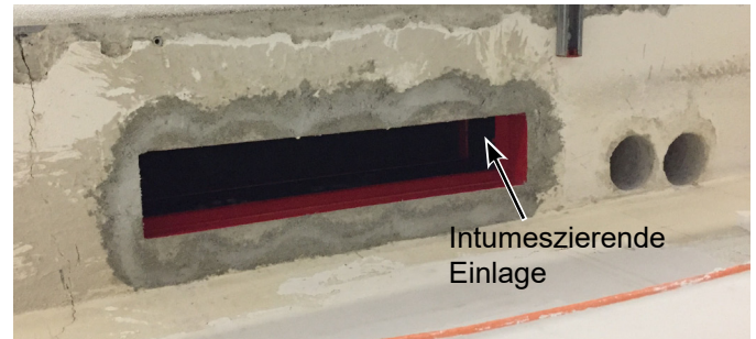
Ansicht von unten der Firebreak Kabelbox eingemörtel in einer Decke vor dem Durchführen der Kabel. Intumeszierende Einlage
