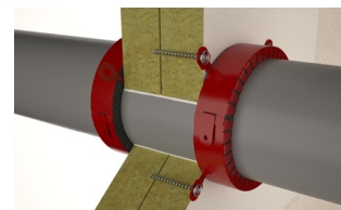
Montage des deux côtés dans la paroi (avec vis en spirale)
