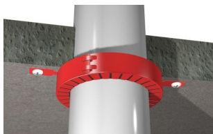
Montage au-dessous du plafond
