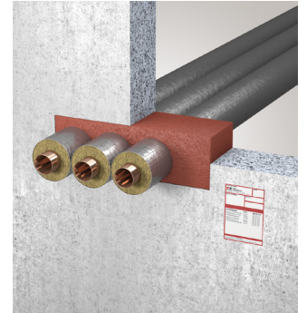
Obturation de tuyaux en cuivre, isolés avec laine minérale
