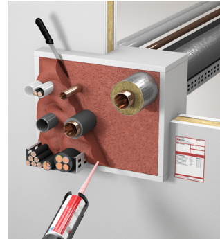
Obturation combinée: occupation max. = 60% de la surface de l'ouverture
