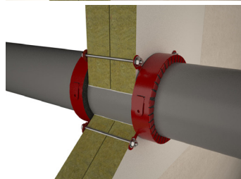
Montage avec tiges filetées M6/M8 (≥ 50 % doivent être fixées, ça veut dire, 2 de 4 ou 3 de 5, réparties également)
