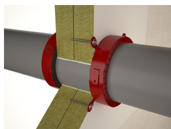
Montage avec vis en spirale (il faut utiliser toutes les languettes)
