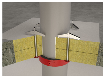
Montage avec chevilles à res- sort I M4 (≥ 50 % doivent être fixées, ça veut dire, 2 de 4 / 3 de 5, réparties également)
