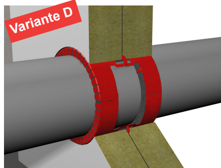
4d. Montagevariante mit eingehängter Brandschutzmanschette. Siehe Seite 2.
