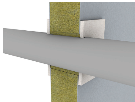
3. Um das Rohr sind Plattenstücke aus 10 mm starken Promatex®-Platten in einer Breite von 50 mm mit 3,5 x 100 mm Schnellbauschrauben zu befestigen.
