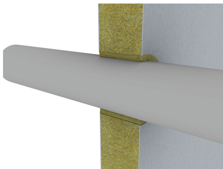
2. Der Ringspalt von max. 10 mm mit einer geeigneten Mineralwolle RF1 (40 kg/m³) füllen und verdichten.
