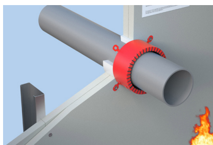
Typ 1 = einseitige Abschottung
