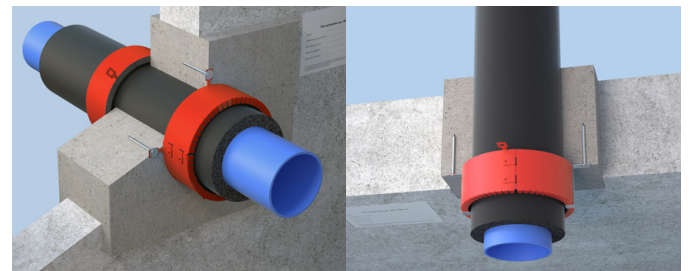
Kunststoffrohr im Mörtelschott Promastop®-M
