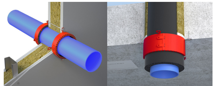
Kunststoffrohr in einer Kernbohrung in der Leichtbauwand, Massivwand oder Massivdecke
