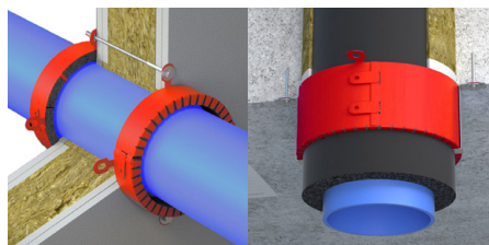
Aufgesetzt
